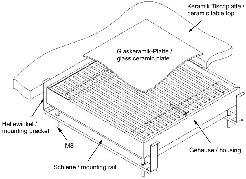
3D Ansicht/ 3D view
