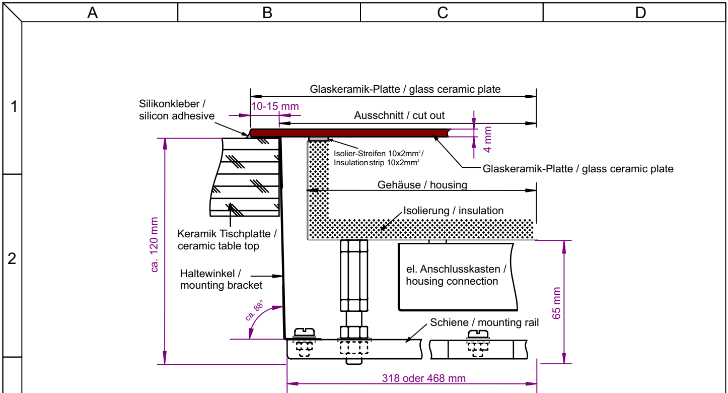
Seitenansicht/ side view
